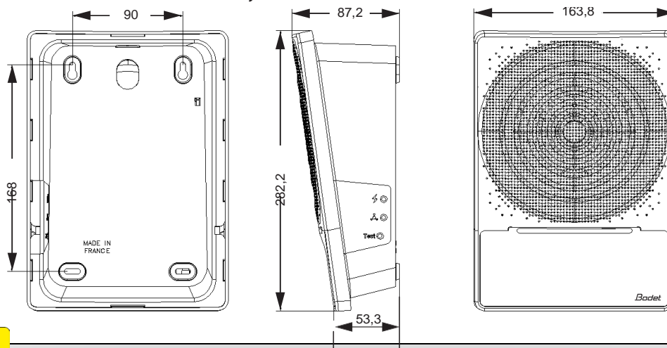
Rozměry v mm
